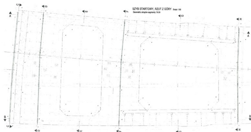
Rys. 6. Rzut z góry na stropy segmentów 19-24 z widocznymi dwoma otworami
