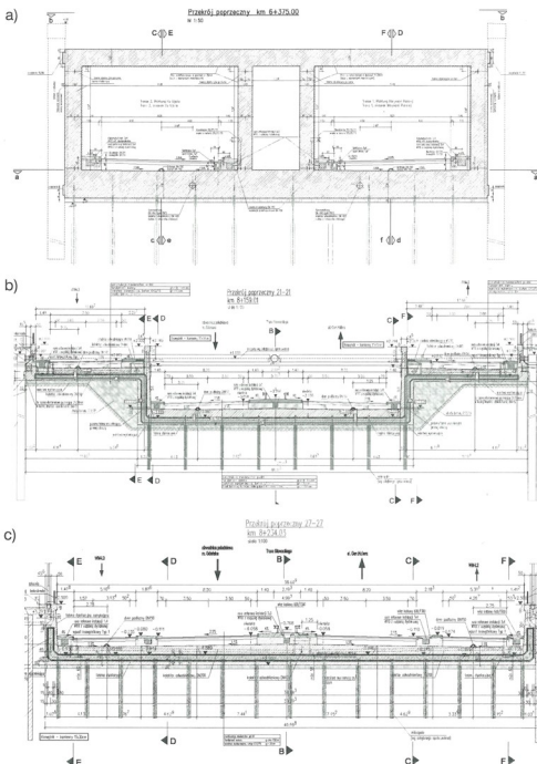
Rys. 2. Przekroje poprzeczne w poszczególnych segmen- tach: a) tunel w wykopie otwartym – segment 17, b) wanna żelbetowa – seg- ment 70, c) wanna żelbetowa – segment 75
