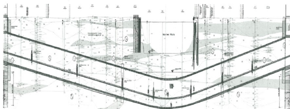
Rys. 4. Przebieg tunelu drążonego
